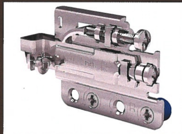
Nieuwe kastophangers van Camar met beveiliging tegen uithaken. © VanOpstal
