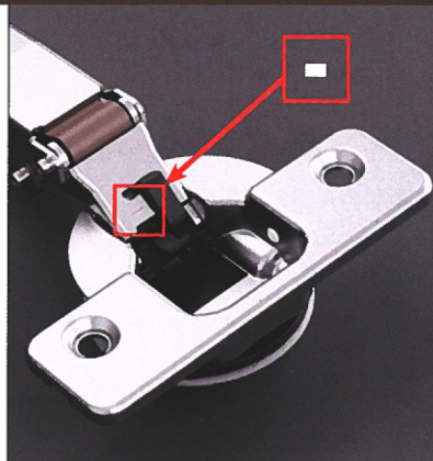
Het nieuwe Silentia+ scharnier van Salice in première voor de Benelux. © VanOpstal
